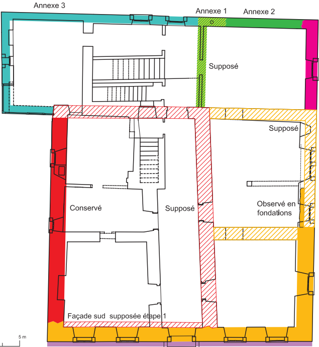
Reconstruction complète de la façade sud aux étapes 2 et 8
